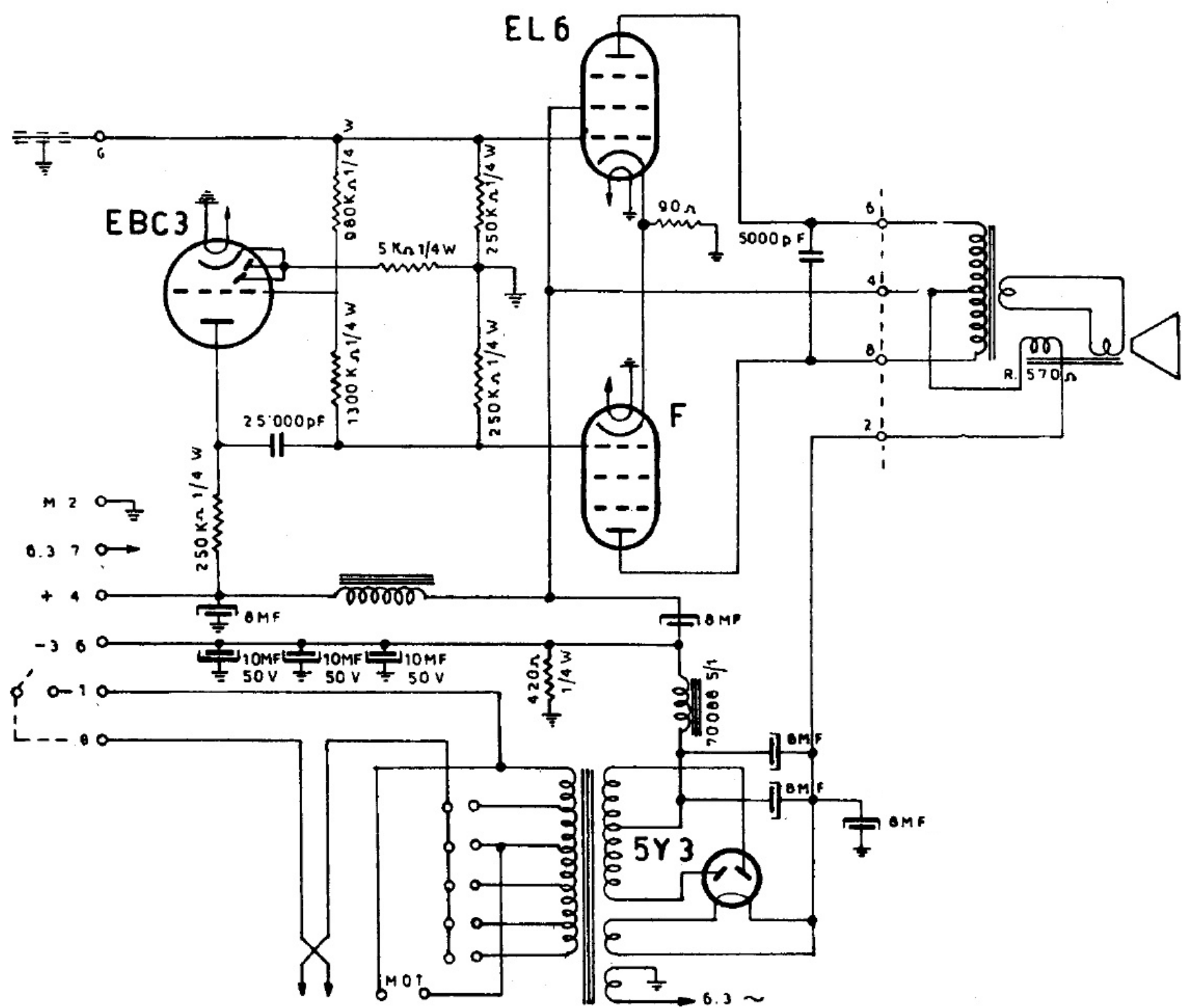
SAVIGLIANO - Mod. OS 710 - Amplificatore finale in contropase e alimentatore anodico. Parte AF/MF stesso circuito e telaio del mod. OS 51. Potenza d'uscita 10 W.
